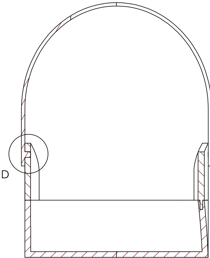
SECTION A-A
